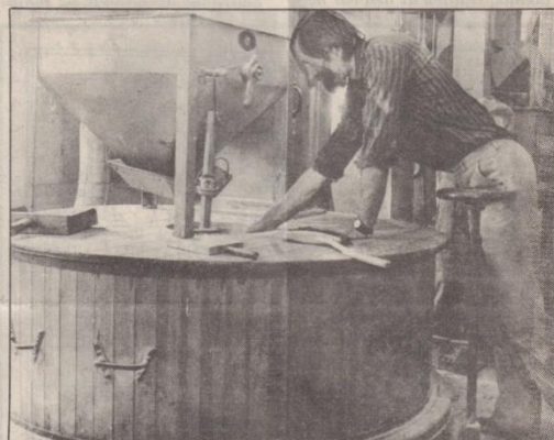
— Här nere roterar kvarnstenen och kornet mals till kornmjöl, visar mjölnare Birger Ledström och kontrollerar att allt är i sin ordning.
